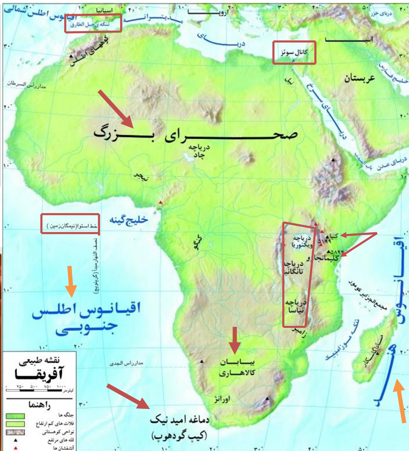
○ آبشار ویکتوریا در اثر فرو ریختن آبهای رود زامبیز در محل یک گسل (شکستگی)، پدید آمده است.
